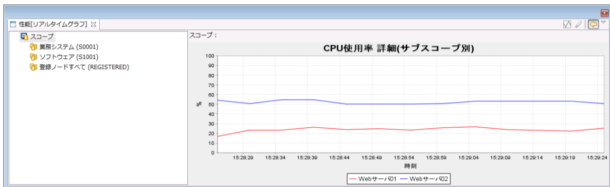
図 12-7 詳細 (サブスコープ別) グラフ
