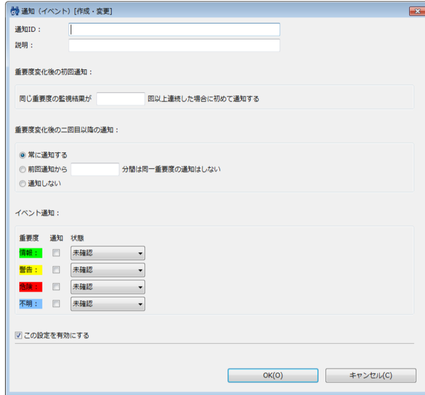
図 5-4 通知（イベント）[作成・変更]ダイアログ
