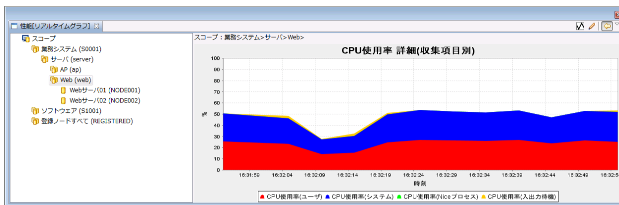
図 12-10 積み上げ面グラフ表示形式
