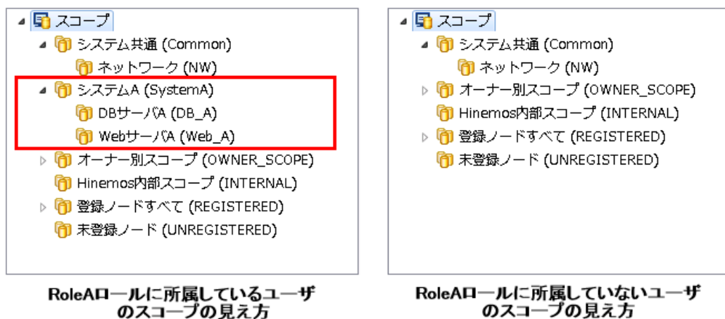
図 12-2 ロールごとのスコープの見え方
