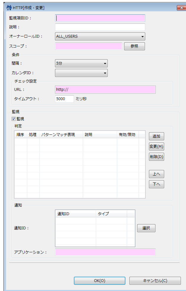
図 7-7 HTTP[作成・変更]ダイアログ (文字列)
