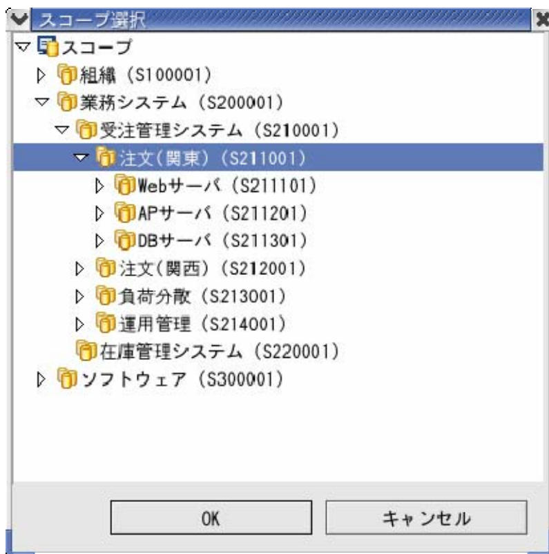
図 12-30 スコープ選択ダイアログ
